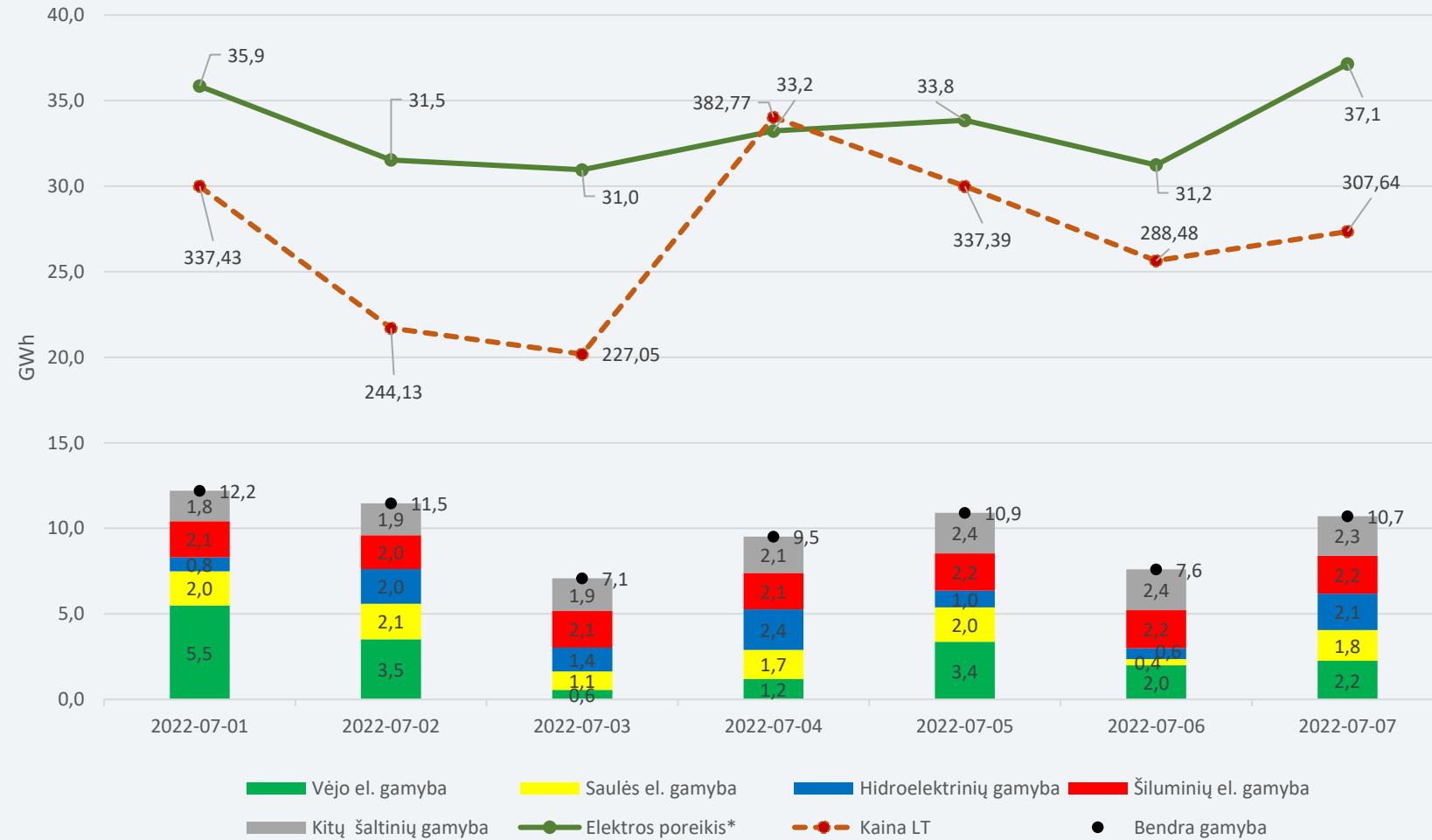
Elektros gamyba Lietuvoje liepos mėn. 1 - 7 d.
