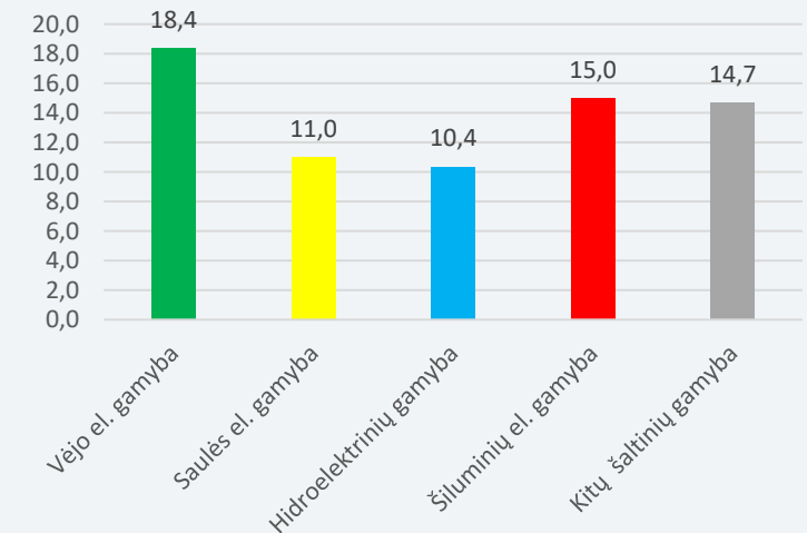
Bendra elektros gamyba liepos 1-7 d. pagal rūšis (GWh)
